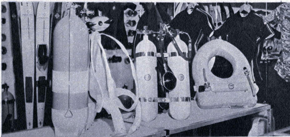
bola con l'erogatore "Corallo" e la bardatura rigida; al centro il "MINIBI" di 8 litri a 180 atmosfere; a destra il salvagente subacqueo di profondità.
