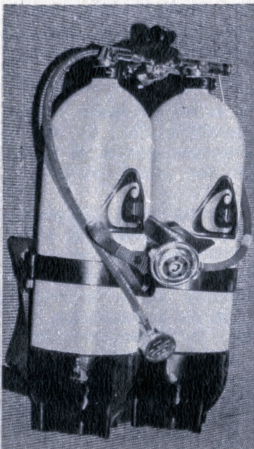
Il gruppo autorespiratore Cressi con rubinetteria a tre attacchi.
