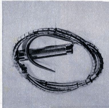
Sotto ed a destra: il raffio tascabile di A. Gengarelli raggiunge in estensione una lunghezza di cm. 85, ripiegato di cm. 11,5x17x1 in astuccio. E' composto di piccole boccole di acciaio con un'anima pure in acciaio. Lire 5.000.
