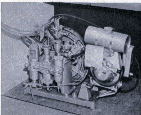
Il compressore "Bauer utilis plus" della Cressi.
