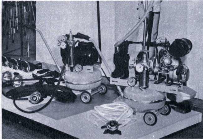
I due compressorini con narghilè presentati dalla Cressi, a sinistra quello elettrico, a destra quello con motore a scoppio.
