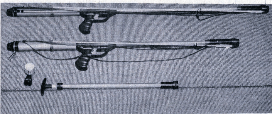
I fucili MACH 0,9 e MACH 0,1 con pompa e manometro di controllo.
